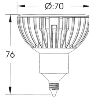
<外形寸法図>
