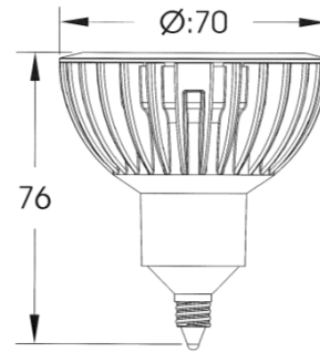
<外形寸法図>
